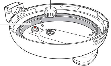
浮き圧力弁
